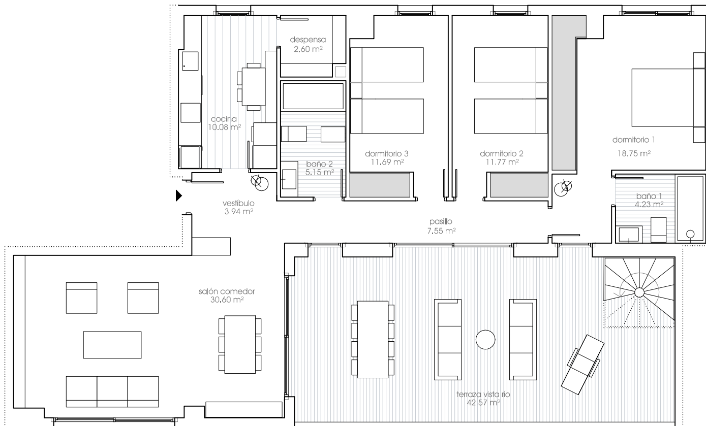
Planta ático
